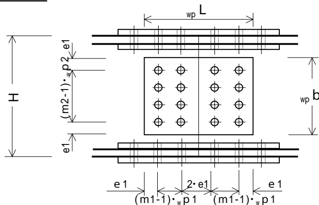
側面図
