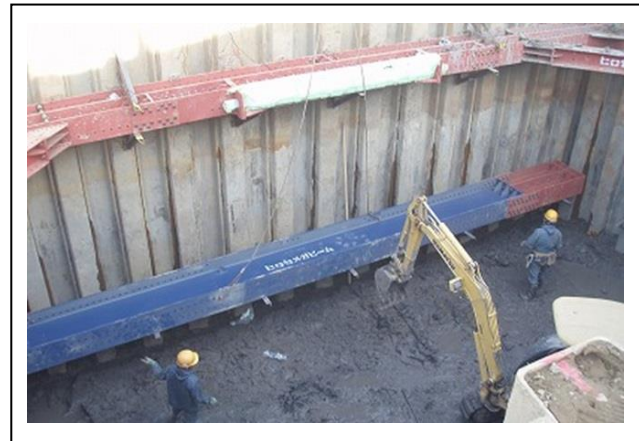
<土木物件> 国土交通省 関東地方整備局 渡良瀬川河川事務所 潮田建設(株) H26 伊保内橋下部工事
